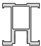
ROČAJ - H (315001)
