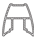
ROČAJ - V (315003)
