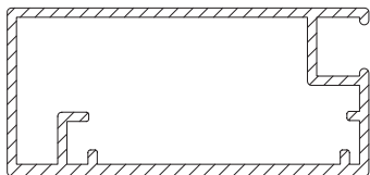
PROFIL - 3820 (312382065)
