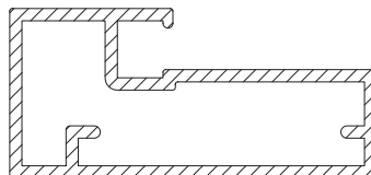
PROFIL - 4520 (312452029)
