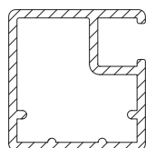
PROFIL - 2001 (312200129)
