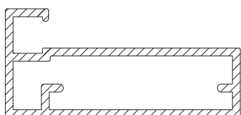
PROFIL - 4508 (312450505)
